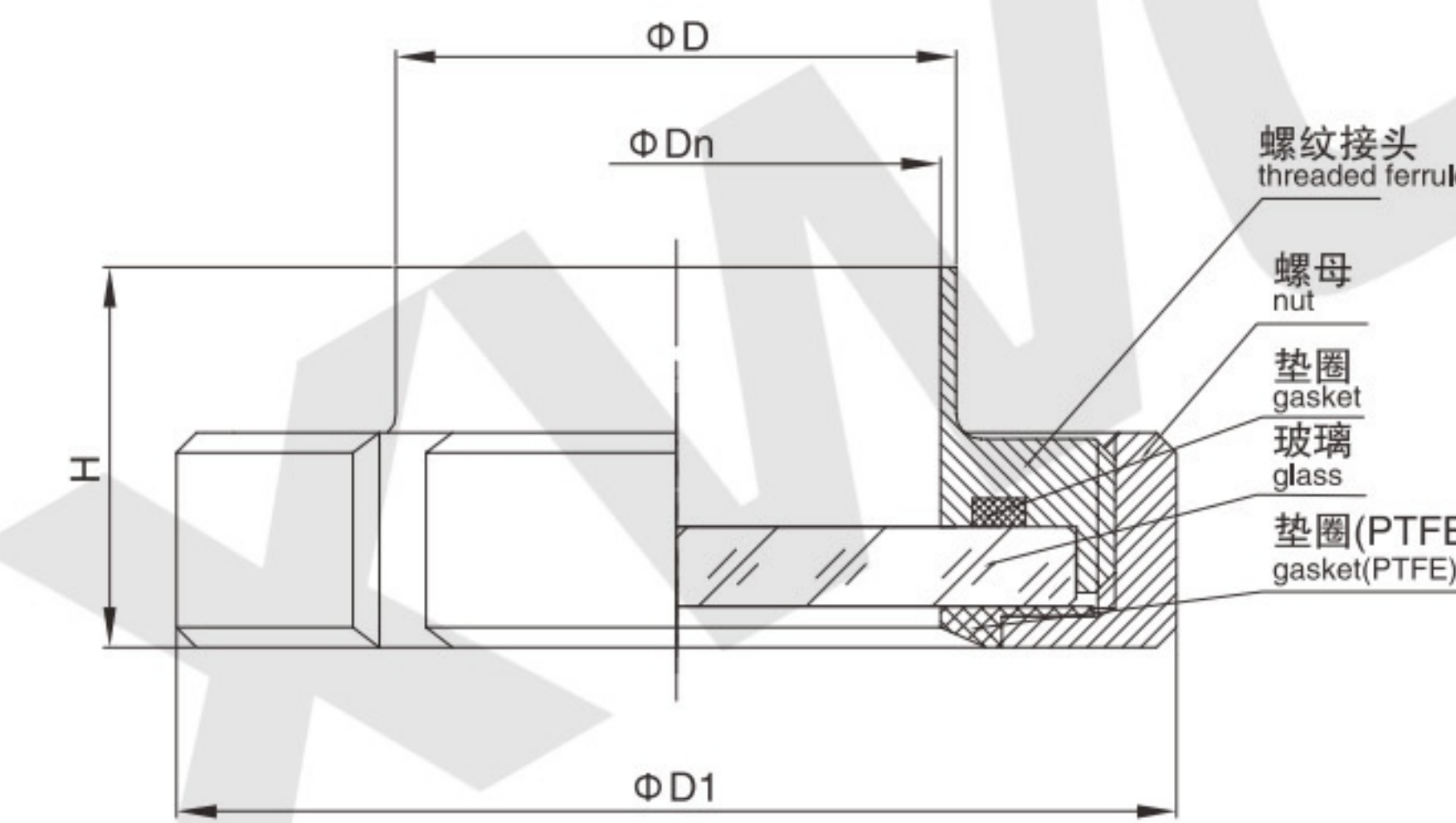
由任视镜(DIN)
